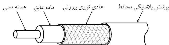
ساختار کابل کوآکسیال
